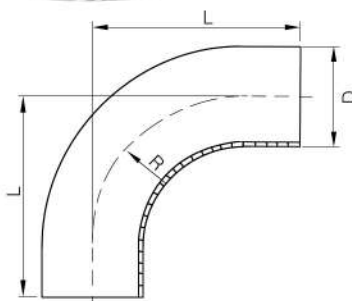
ELBOW 90° LONG TANGENT
