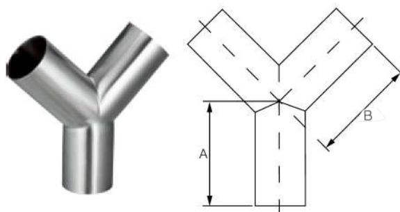
WELDED TEE Y TRUE 28WB
